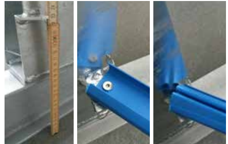
Einbautiefe des Stahlträgers (ca. 22,5 cm)
