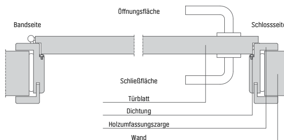
Zargenumrüstset (aus einer Standardzarge wird eine Wohnungsabschluszzarge)
